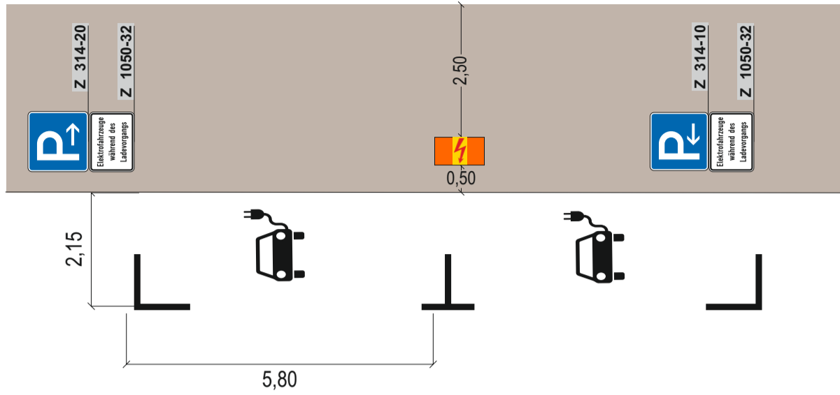
Bild 1: Längsaufstellung
