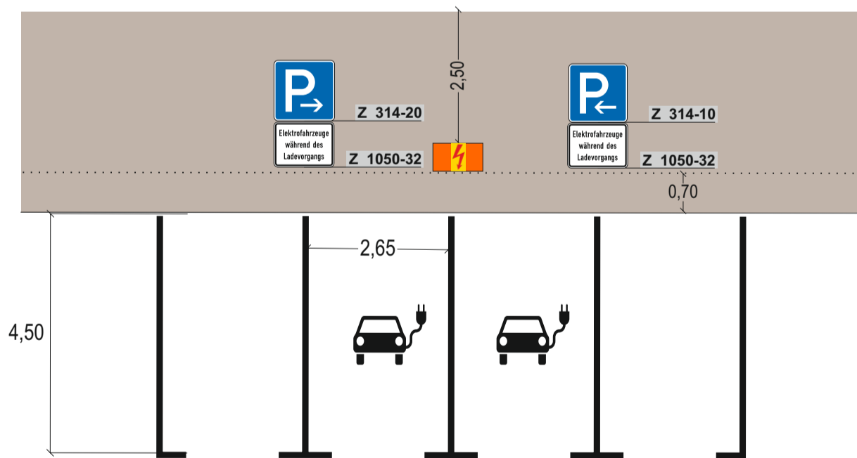
Bild 3: Senkrechtaufstellung
