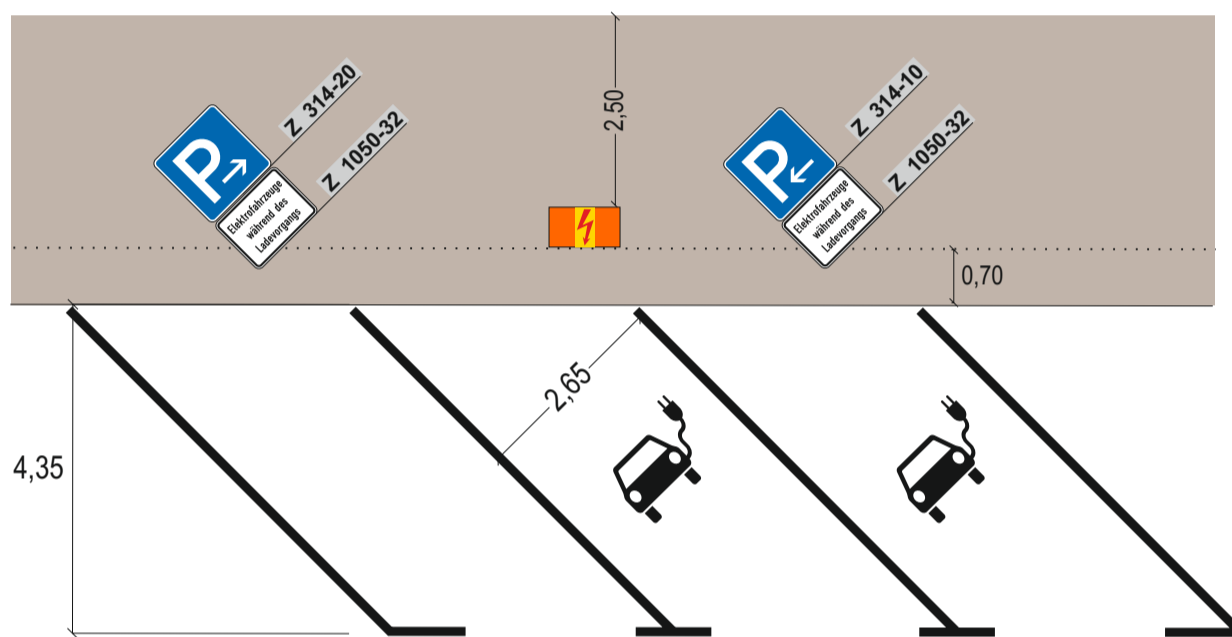
Bild 2: Schrägaufstellung 45 Grad
